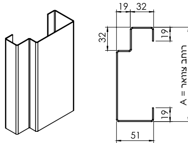
משקוף דגם C (ניתן להזמין עם/בלי הלבשות קליק)
